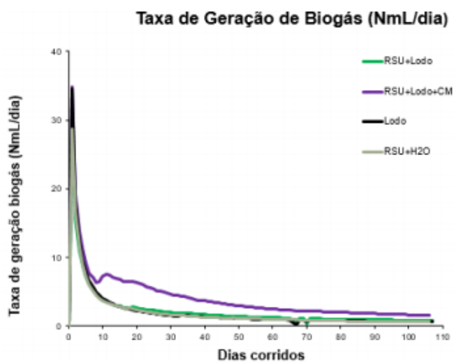
Figura 5 – Taxa de geração de biogás (NmL/dia). Onde: RSU (resíduo sólido urbano); H 2 O (água); CM (consórcio microbiológico) = (consórcio bacteriano).
