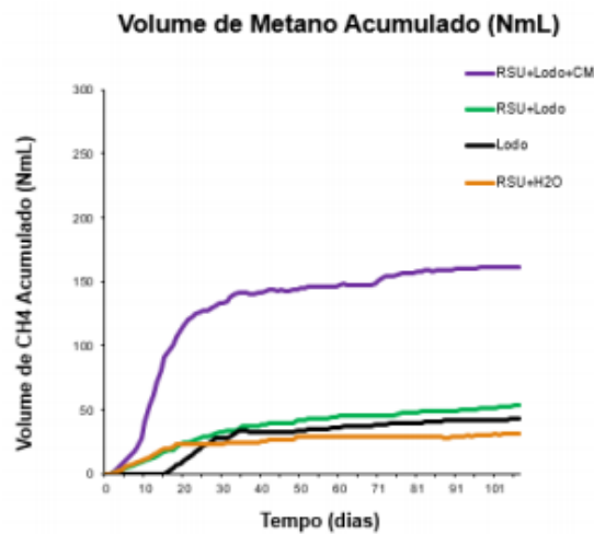
Figura 8. Volume de metano acumulado (NmL). Onde: RSU (resíduo sólido urbano); H 2 O (água); CM (Consórcio Microbiológico = Consórcio Bacteriano). Fonte: Adaptado de HOLANDA (2016).
