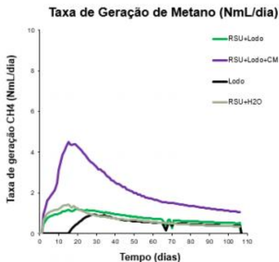
Figura 6 - Taxa de geração de metano (NmL/dia). Onde: RSU (Resíduo Sólido Urbano); H 2 O (água); CM (Consórcio Microbiológico = Consórcio Bacteriano). Fonte: Adaptado de HOLANDA (2016).
