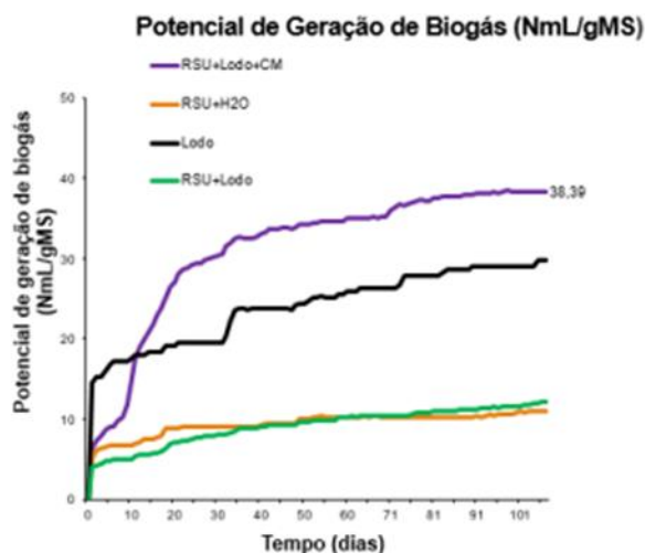
Figura 9 – Potencial de geração de biogás (NmL/gMS). Onde: RSU (resíduo sólido urbano); H 2 O (água); CM (Consórcio Microbiológico = Consórcio Bacteriano) Fonte: Adaptado de HOLANDA (2016).
