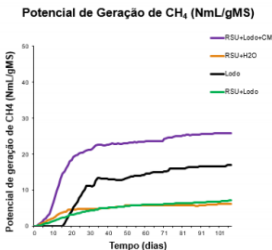
Figura 10 – Potencial de geração de metano (NmL/gMS). Onde: RSU (resíduo sólido urbano); H 2 O (água); CM (Consórcio Microbiológico = Consórcio Bacteriano). Fonte: Adaptado de HOLANDA (2016).
