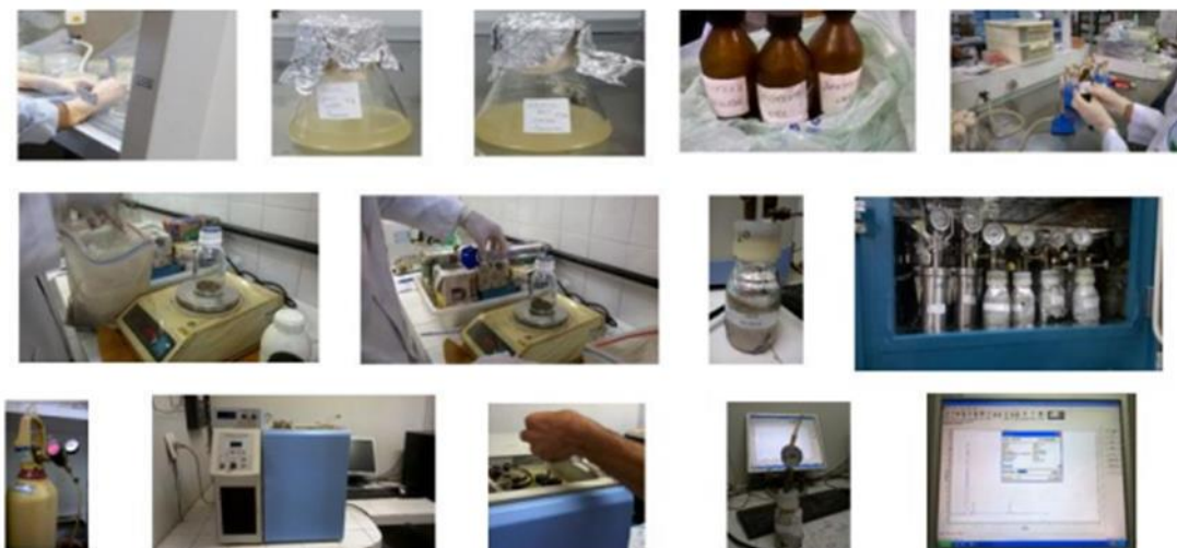
Figura 4 – Etapas dos processos de desenvolvimento do consórcio de microrganismos, inoculação nos biorreatores BMP, monitoramento e análise quantitativa dos gases metano e dióxido de carbono presentes. Fonte: MÉLO-SCHLUB (2016).
