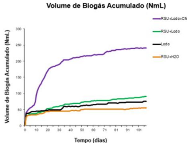
Figura 7. Volume de biogás acumulado (NmL). Onde: RSU (resíduo sólido urbano); H 2 O (água); CM (Consórcio Microbiológico = Consórcio Bacteriano) Fonte: Adaptado de HOLANDA (2016).
